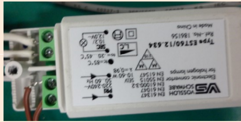
할로겐용 안정기
